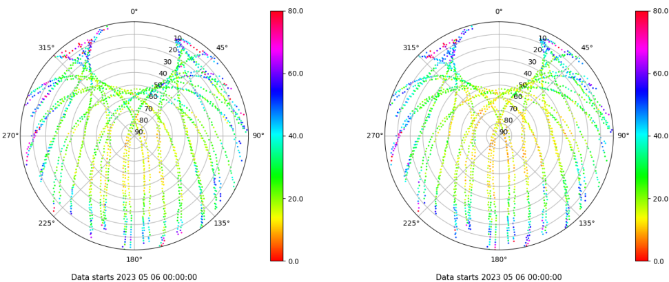
Skyplot for station ZFRA. Parameter M1C Data file ZFRA00ESP_R_2023126.xtr Skyplot for station ZFRA. Parameter M2P Data file ZFRA00ESP_R_2023126.xtr
