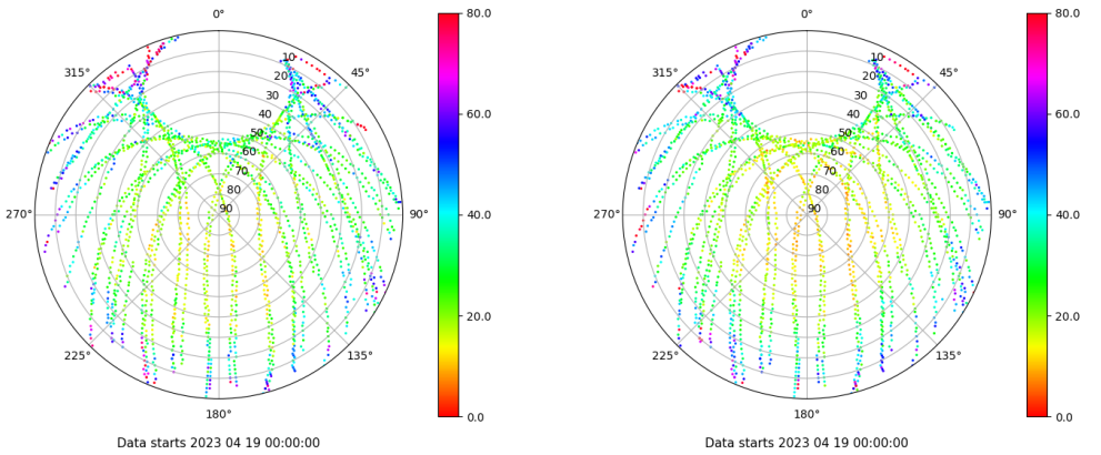
Skyplot for station ZFRA. Parameter M1C Data file ZFRA00ESP_R_2023109.xtr Skyplot for station ZFRA. Parameter M2P Data file ZFRA00ESP_R_2023109.xtr
