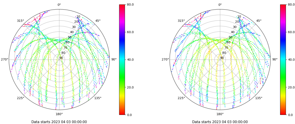
Skyplot for station ZFRA. Parameter M1C Data file ZFRA00ESP_R_2023093.xtr Skyplot for station ZFRA. Parameter M2P Data file ZFRA00ESP_R_2023093.xtr
