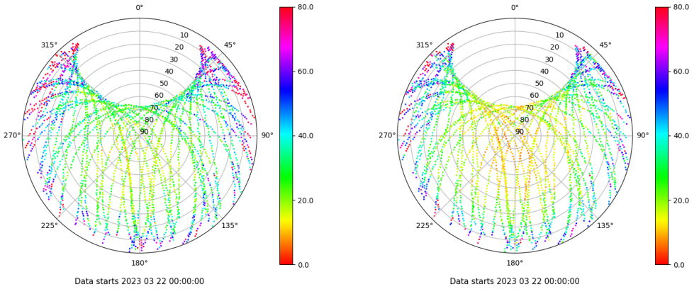
Skyplot for station ZFRA. Parameter M1C Data file ZFRA00ESP_R_2023081.xtr Skyplot for station ZFRA. Parameter M2W Data file ZFRA00ESP_R_2023081.xtr
