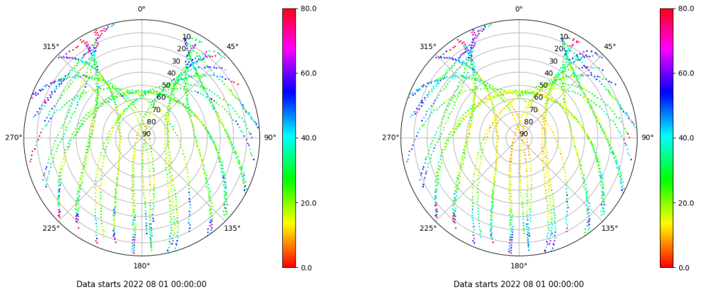
Skyplot for station ZFRA. Parameter M1C Data file ZFRA00ESP_R_2022213.xtr Skyplot for station ZFRA. Parameter M2P Data file ZFRA00ESP_R_2022213.xtr
