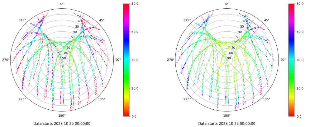
Skyplot for station ZARA. Parameter M1C Data file ZARA00ESP_R_2023298.xtr Skyplot for station ZARA. Parameter M2C Data file ZARA00ESP_R_2023298.xtr
