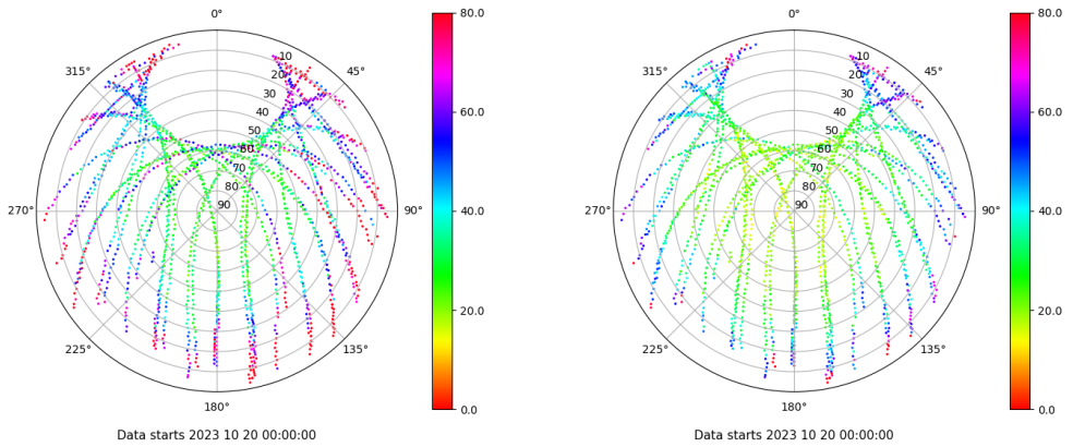
Skyplot for station ZARA. Parameter M1C Data file ZARA00ESP_R_2023293.xtr Skyplot for station ZARA. Parameter M2C Data file ZARA00ESP_R_2023293.xtr
