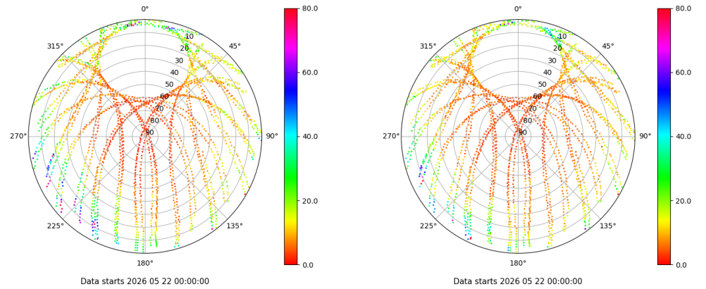
Skyplot for station XIXO. Parameter M1C Data file XIXO00ESP_R_2026142.xtr Skyplot for station XIXO. Parameter M2C Data file XIXO00ESP_R_2026142.xtr
