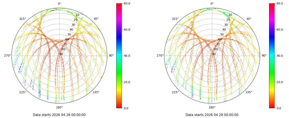
Skyplot for station XIXO. Parameter M1C Data file XIXO00ESP_R_2026118.xtr Skyplot for station XIXO. Parameter M2C Data file XIXO00ESP_R_2026118.xtr
