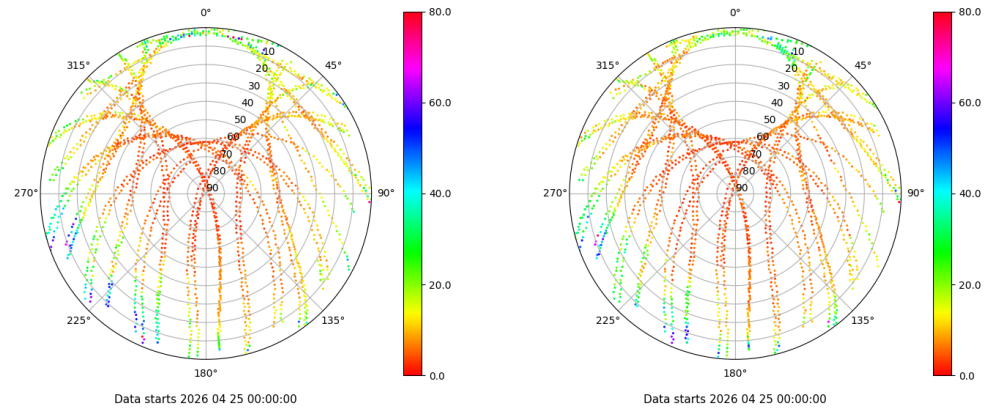
Skyplot for station XIXO. Parameter M1C Data file XIXO00ESP_R_2026115.xtr Skyplot for station XIXO. Parameter M2C Data file XIXO00ESP_R_2026115.xtr
