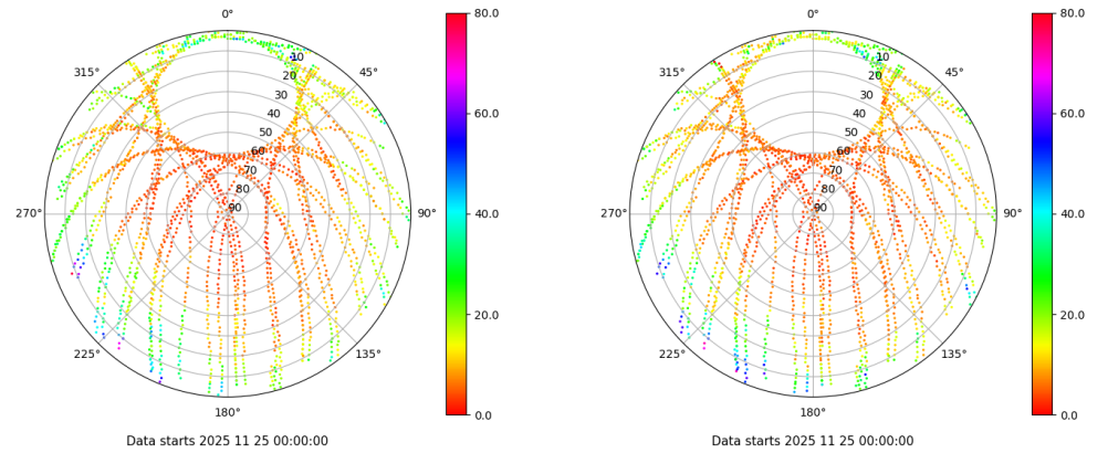
Skyplot for station XIXO. Parameter M1C Data file XIXO00ESP_R_2025329.xtr Skyplot for station XIXO. Parameter M2C Data file XIXO00ESP_R_2025329.xtr
