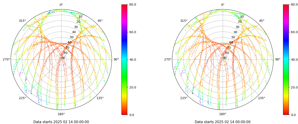
Skyplot for station XIXO. Parameter M1C Data file XIXO00ESP_R_2025045.xtr Skyplot for station XIXO. Parameter M2C Data file XIXO00ESP_R_2025045.xtr
