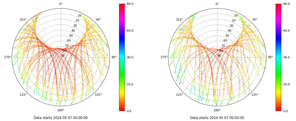
Skyplot for station XIXO. Parameter M1C Data file XIXO00ESP_R_2024128.xtr Skyplot for station XIXO. Parameter M2S Data file XIXO00ESP_R_2024128.xtr
