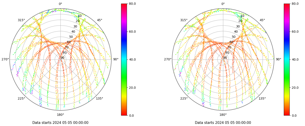
Skyplot for station XIXO. Parameter M1C Data file XIXO00ESP_R_2024126.xtr Skyplot for station XIXO. Parameter M2C Data file XIXO00ESP_R_2024126.xtr
