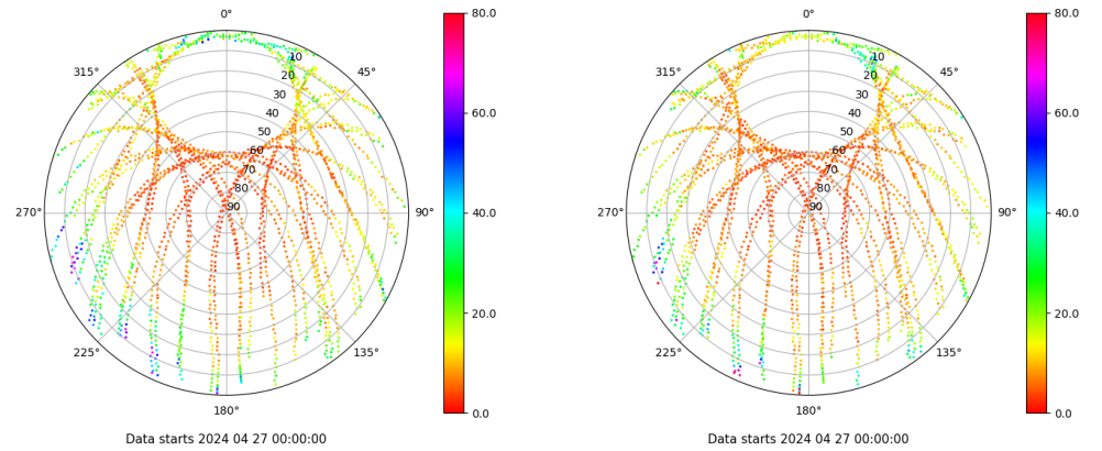
Skyplot for station XIXO. Parameter M1C Data file XIXO00ESP_R_2024118.xtr Skyplot for station XIXO. Parameter M2C Data file XIXO00ESP_R_2024118.xtr
