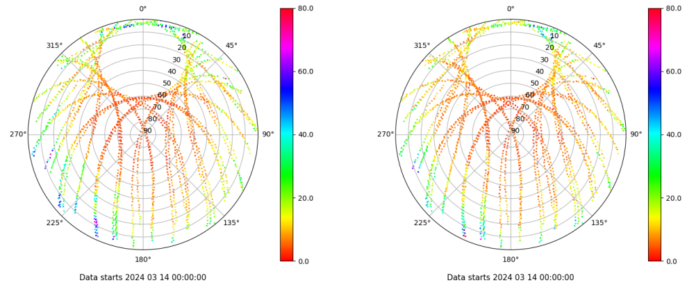
Skyplot for station XIXO. Parameter M1C Data file XIXO00ESP_R_2024074.xtr Skyplot for station XIXO. Parameter M2C Data file XIXO00ESP_R_2024074.xtr
