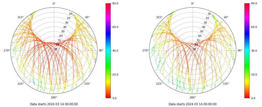
Skyplot for station XIXO. Parameter M1C Data file XIXO00ESP_R_2024074.xtr Skyplot for station XIXO. Parameter M2S Data file XIXO00ESP_R_2024074.xtr
