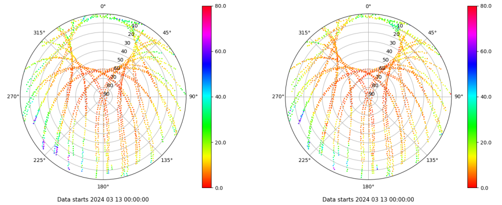
Skyplot for station XIXO. Parameter M1C Data file XIXO00ESP_R_2024073.xtr Skyplot for station XIXO. Parameter M2C Data file XIXO00ESP_R_2024073.xtr
