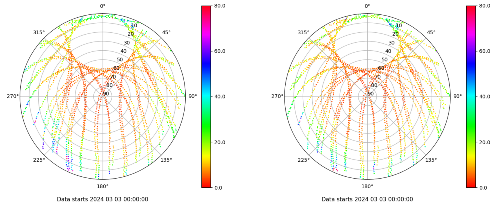
Skyplot for station XIXO. Parameter M1C Data file XIXO00ESP_R_2024063.xtr Skyplot for station XIXO. Parameter M2C Data file XIXO00ESP_R_2024063.xtr
