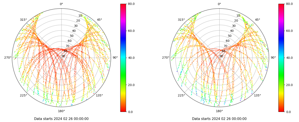
Skyplot for station XIXO. Parameter M1C Data file XIXO00ESP_R_2024057.xtr Skyplot for station XIXO. Parameter M2S Data file XIXO00ESP_R_2024057.xtr
