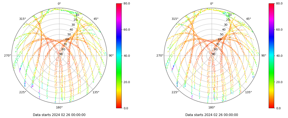
Skyplot for station XIXO. Parameter M1C Data file XIXO00ESP_R_2024057.xtr Skyplot for station XIXO. Parameter M2C Data file XIXO00ESP_R_2024057.xtr
