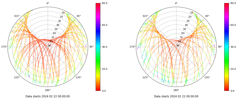
Skyplot for station XIXO. Parameter M1C Data file XIXO00ESP_R_2024053.xtr Skyplot for station XIXO. Parameter M2S Data file XIXO00ESP_R_2024053.xtr
