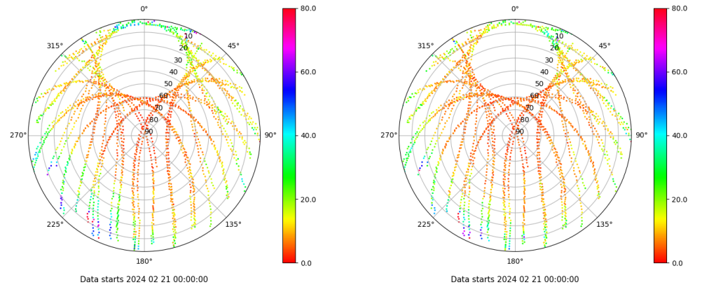
Skyplot for station XIXO. Parameter M1C Data file XIXO00ESP_R_2024052.xtr Skyplot for station XIXO. Parameter M2C Data file XIXO00ESP_R_2024052.xtr
