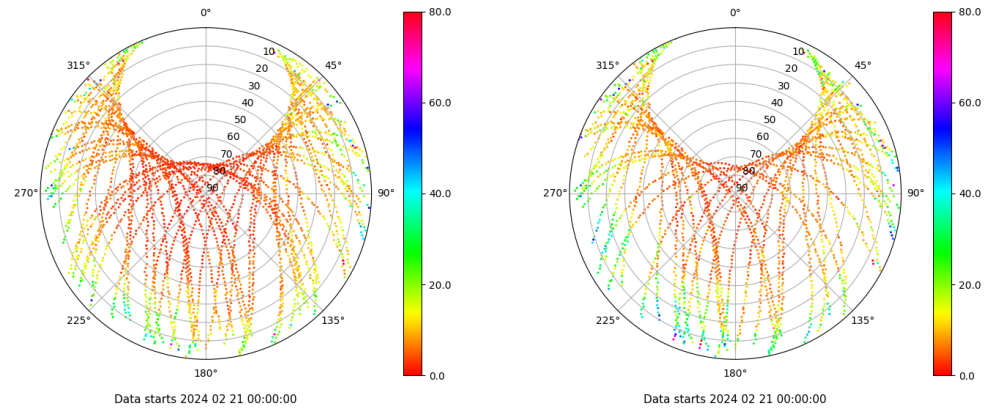
Skyplot for station XIXO. Parameter M1C Data file XIXO00ESP_R_2024052.xtr Skyplot for station XIXO. Parameter M2S Data file XIXO00ESP_R_2024052.xtr
