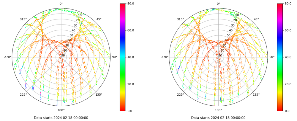
Skyplot for station XIXO. Parameter M1C Data file XIXO00ESP_R_2024049.xtr Skyplot for station XIXO. Parameter M2C Data file XIXO00ESP_R_2024049.xtr
