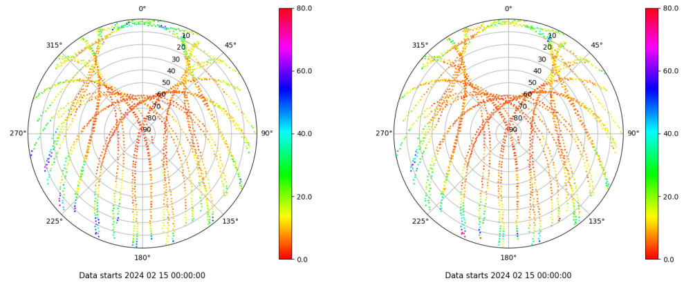
Skyplot for station XIXO. Parameter M1C Data file XIXO00ESP_R_2024046.xtr Skyplot for station XIXO. Parameter M2C Data file XIXO00ESP_R_2024046.xtr
