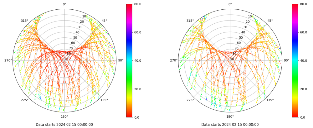
Skyplot for station XIXO. Parameter M1C Data file XIXO00ESP_R_2024046.xtr Skyplot for station XIXO. Parameter M2S Data file XIXO00ESP_R_2024046.xtr
