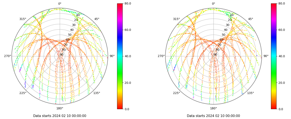
Skyplot for station XIXO. Parameter M1C Data file XIXO00ESP_R_2024041.xtr Skyplot for station XIXO. Parameter M2C Data file XIXO00ESP_R_2024041.xtr
