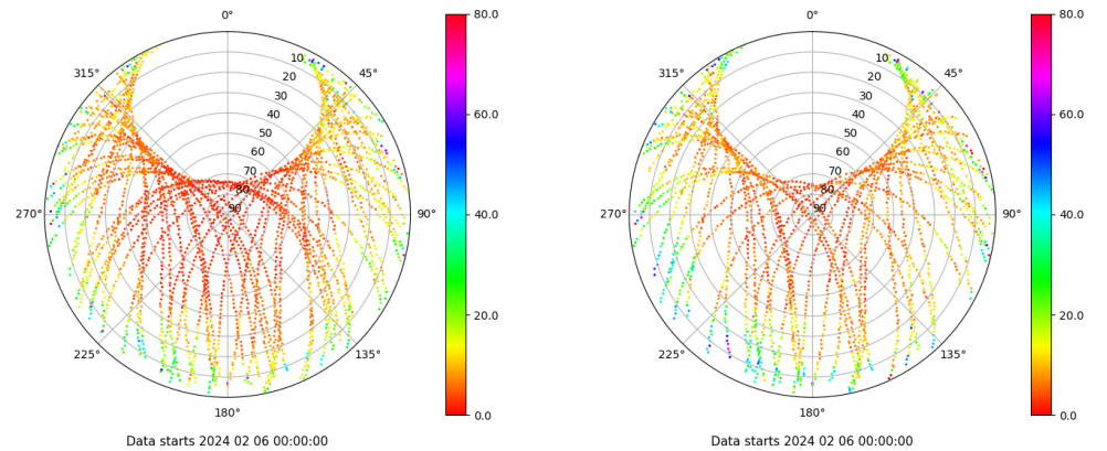
Skyplot for station XIXO. Parameter M1C Data file XIXO00ESP_R_2024037.xtr Skyplot for station XIXO. Parameter M2S Data file XIXO00ESP_R_2024037.xtr
