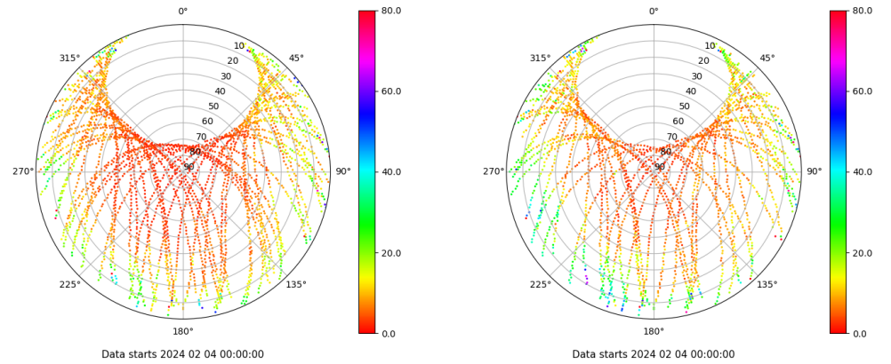
Skyplot for station XIXO. Parameter M1C Data file XIXO00ESP_R_2024035.xtr Skyplot for station XIXO. Parameter M2S Data file XIXO00ESP_R_2024035.xtr
