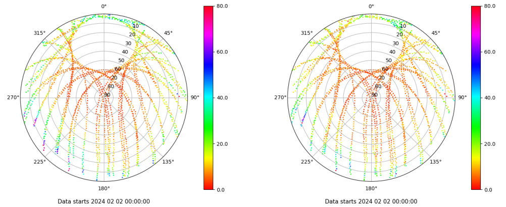
Skyplot for station XIXO. Parameter M1C Data file XIXO00ESP_R_2024033.xtr Skyplot for station XIXO. Parameter M2C Data file XIXO00ESP_R_2024033.xtr
