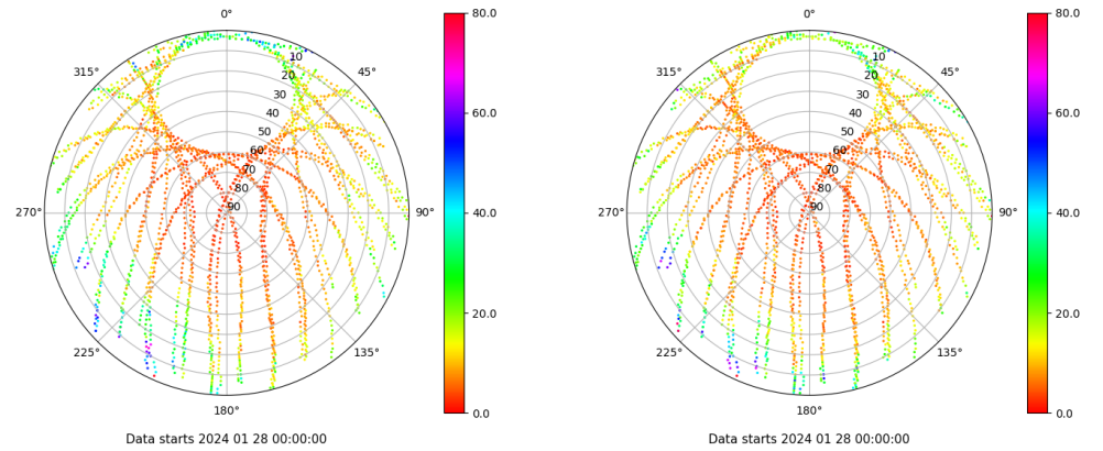
Skyplot for station XIXO. Parameter M1C Data file XIXO00ESP_R_2024028.xtr Skyplot for station XIXO. Parameter M2C Data file XIXO00ESP_R_2024028.xtr
