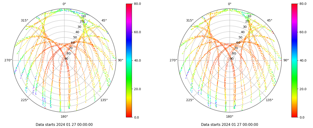
Skyplot for station XIXO. Parameter M1C Data file XIXO00ESP_R_2024027.xtr Skyplot for station XIXO. Parameter M2C Data file XIXO00ESP_R_2024027.xtr
