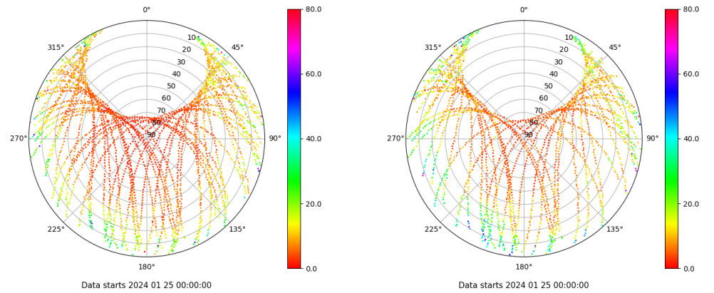
Skyplot for station XIXO. Parameter M1C Data file XIXO00ESP_R_2024025.xtr Skyplot for station XIXO. Parameter M2S Data file XIXO00ESP_R_2024025.xtr
