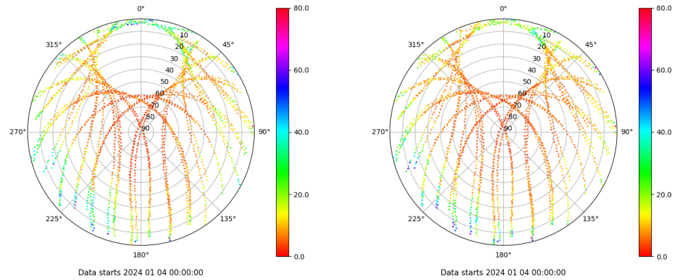
Skyplot for station XIXO. Parameter M1C Data file XIXO00ESP_R_2024004.xtr Skyplot for station XIXO. Parameter M2C Data file XIXO00ESP_R_2024004.xtr
