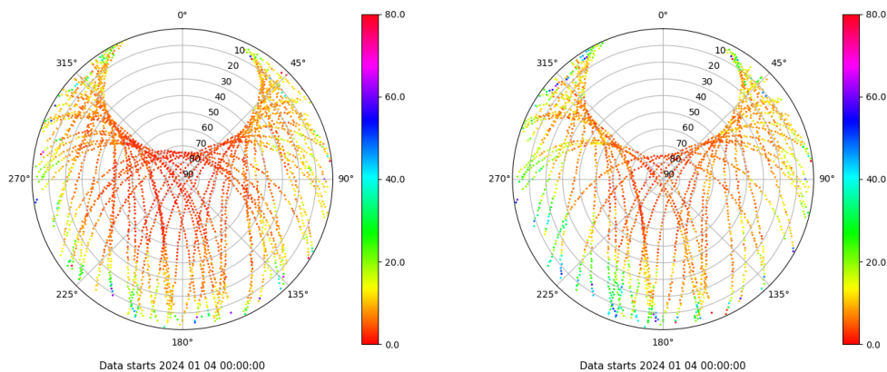
Skyplot for station XIXO. Parameter M1C Data file XIXO00ESP_R_2024004.xtr Skyplot for station XIXO. Parameter M2S Data file XIXO00ESP_R_2024004.xtr
