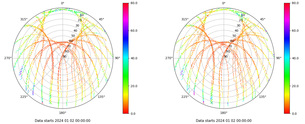
Skyplot for station XIXO. Parameter M1C Data file XIXO00ESP_R_2024002.xtr Skyplot for station XIXO. Parameter M2C Data file XIXO00ESP_R_2024002.xtr
