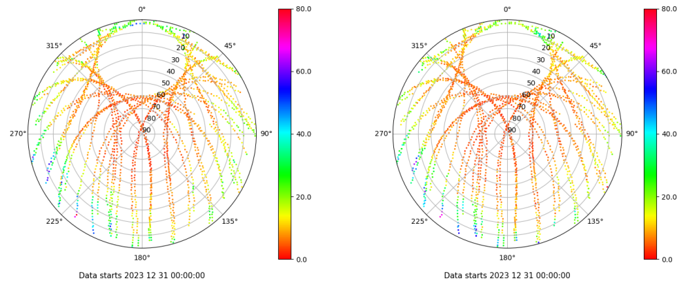
Skyplot for station XIXO. Parameter M1C Data file XIXO00ESP_R_2023365.xtr Skyplot for station XIXO. Parameter M2C Data file XIXO00ESP_R_2023365.xtr
