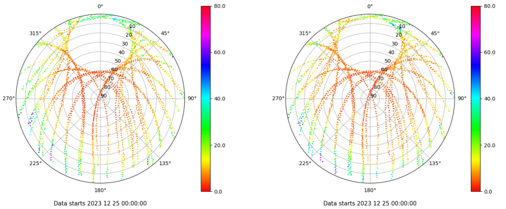
Skyplot for station XIXO. Parameter M1C Data file XIXO00ESP_R_2023359.xtr Skyplot for station XIXO. Parameter M2C Data file XIXO00ESP_R_2023359.xtr
