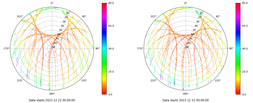
Skyplot for station XIXO. Parameter M1C Data file XIXO00ESP_R_2023356.xtr Skyplot for station XIXO. Parameter M2C Data file XIXO00ESP_R_2023356.xtr
