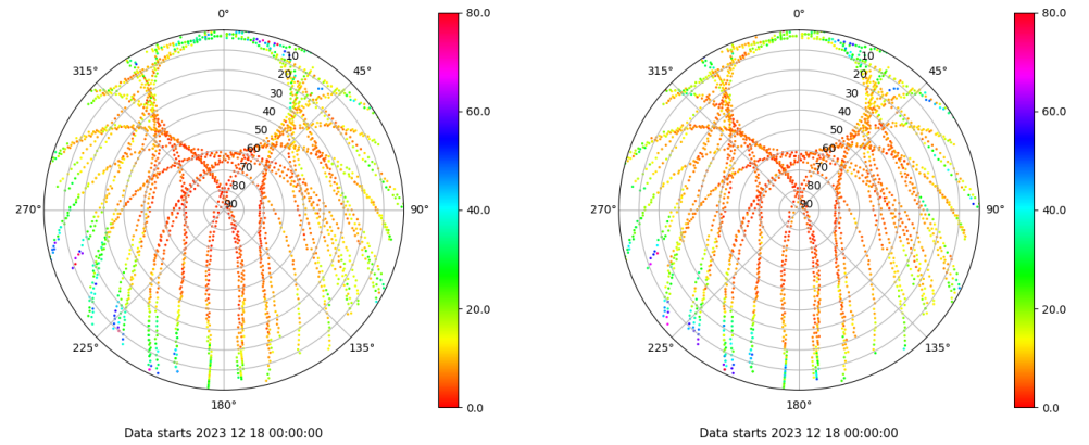
Skyplot for station XIXO. Parameter M1C Data file XIXO00ESP_R_2023352.xtr Skyplot for station XIXO. Parameter M2C Data file XIXO00ESP_R_2023352.xtr
