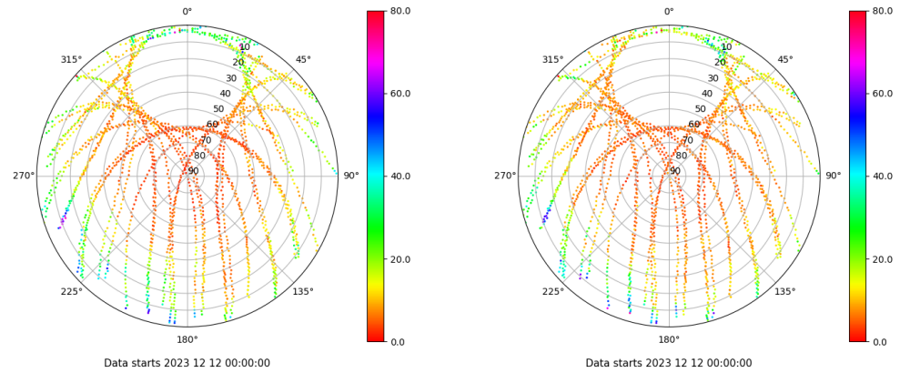
Skyplot for station XIXO. Parameter M1C Data file XIXO00ESP_R_2023346.xtr Skyplot for station XIXO. Parameter M2C Data file XIXO00ESP_R_2023346.xtr
