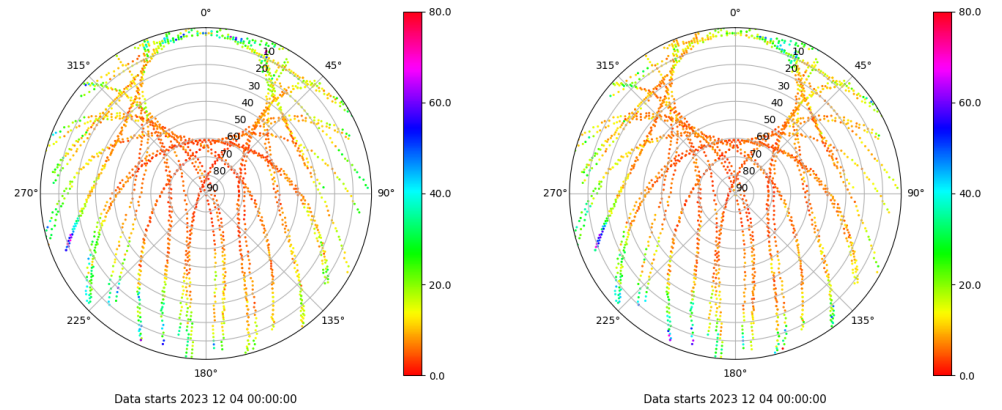
Skyplot for station XIXO. Parameter M1C Data file XIXO00ESP_R_2023338.xtr Skyplot for station XIXO. Parameter M2C Data file XIXO00ESP_R_2023338.xtr
