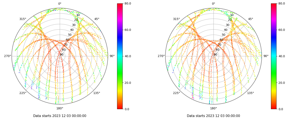
Skyplot for station XIXO. Parameter M1C Data file XIXO00ESP_R_2023337.xtr Skyplot for station XIXO. Parameter M2C Data file XIXO00ESP_R_2023337.xtr
