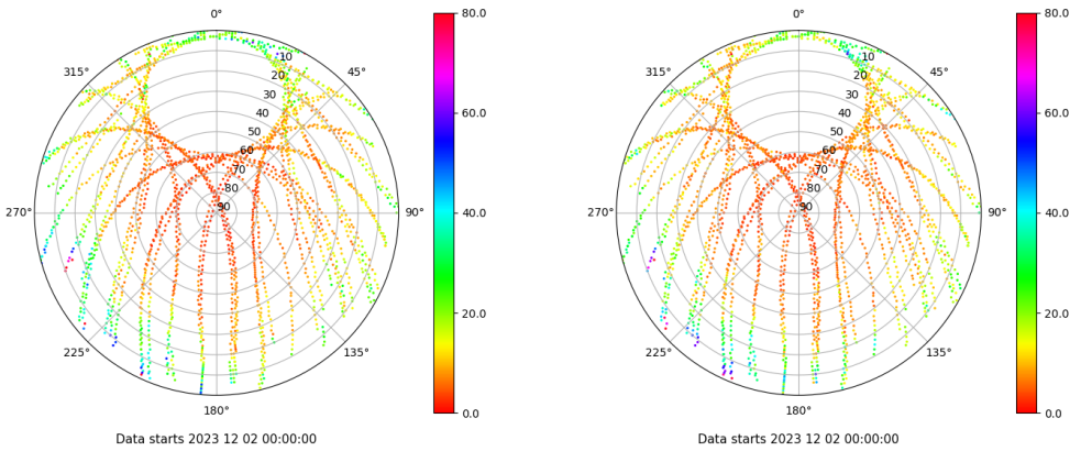
Skyplot for station XIXO. Parameter M1C Data file XIXO00ESP_R_2023336.xtr Skyplot for station XIXO. Parameter M2C Data file XIXO00ESP_R_2023336.xtr
