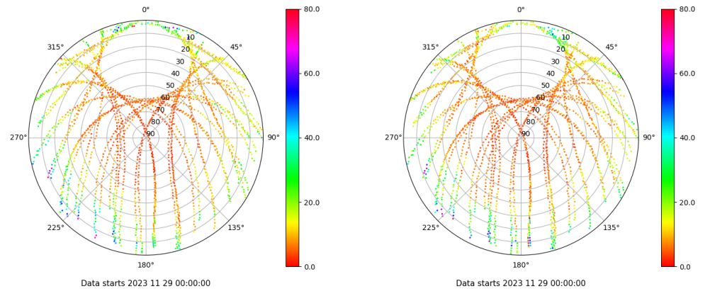
Skyplot for station XIXO. Parameter M1C Data file XIXO00ESP_R_2023333.xtr Skyplot for station XIXO. Parameter M2C Data file XIXO00ESP_R_2023333.xtr
