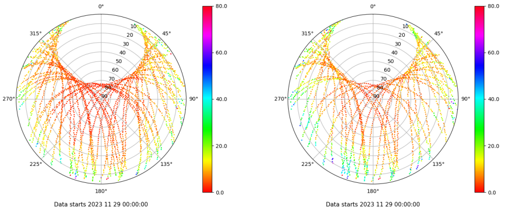
Skyplot for station XIXO. Parameter M1C Data file XIXO00ESP_R_2023333.xtr Skyplot for station XIXO. Parameter M2S Data file XIXO00ESP_R_2023333.xtr
