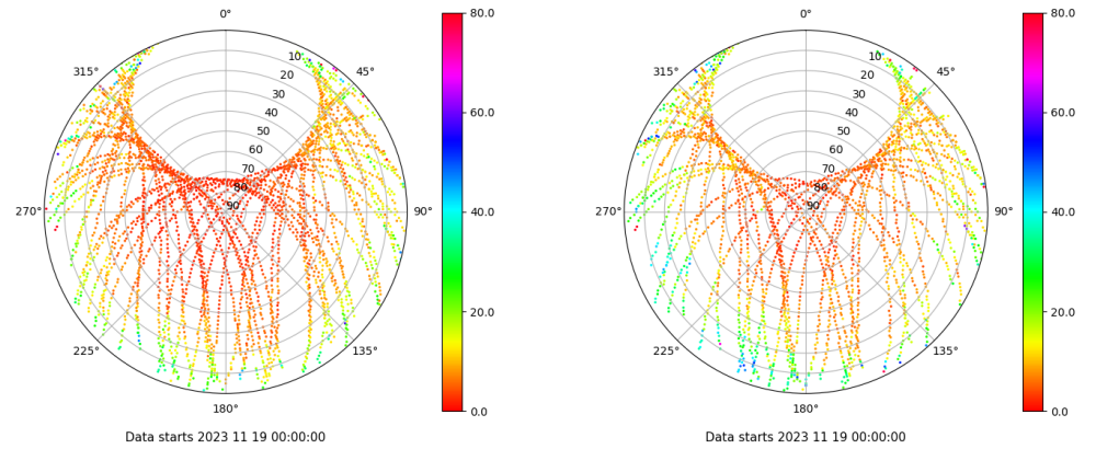
Skyplot for station XIXO. Parameter M1C Data file XIXO00ESP_R_2023323.xtr Skyplot for station XIXO. Parameter M2S Data file XIXO00ESP_R_2023323.xtr
