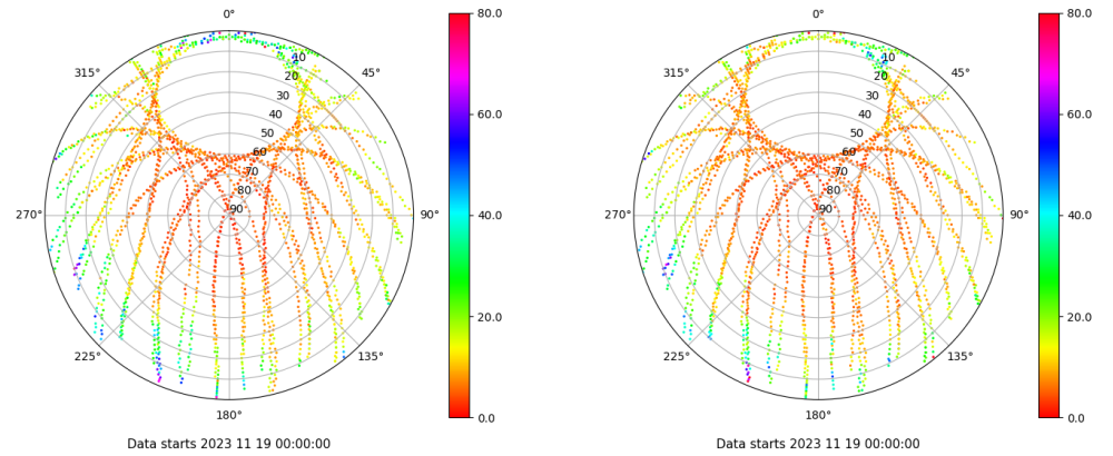
Skyplot for station XIXO. Parameter M1C Data file XIXO00ESP_R_2023323.xtr Skyplot for station XIXO. Parameter M2C Data file XIXO00ESP_R_2023323.xtr
