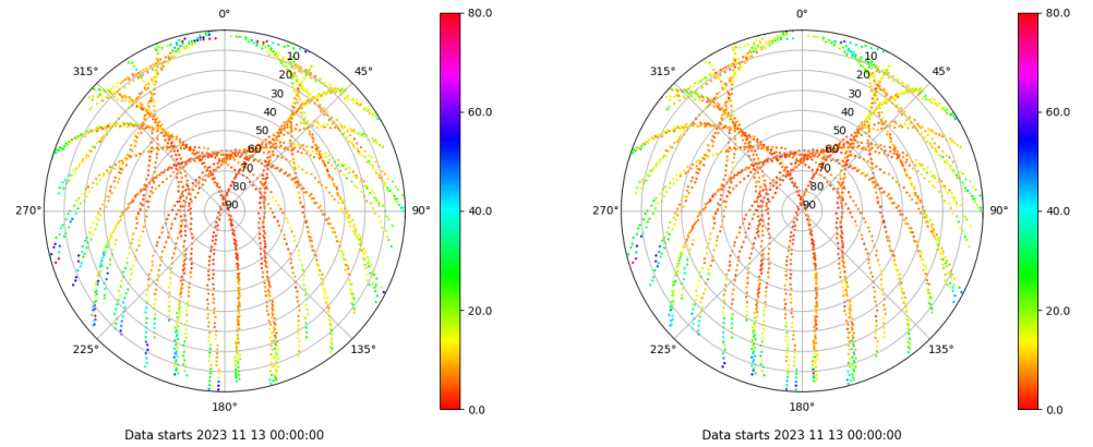
Skyplot for station XIXO. Parameter M1C Data file XIXO00ESP_R_2023317.xtr Skyplot for station XIXO. Parameter M2C Data file XIXO00ESP_R_2023317.xtr
