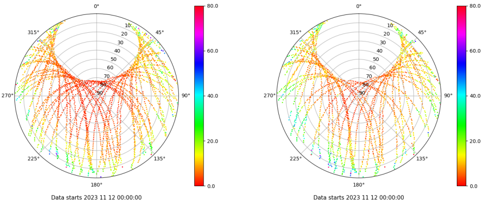
Skyplot for station XIXO. Parameter M1C Data file XIXO00ESP_R_2023316.xtr Skyplot for station XIXO. Parameter M2S Data file XIXO00ESP_R_2023316.xtr
