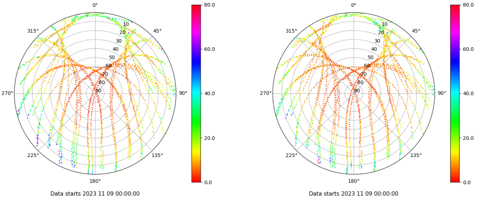
Skyplot for station XIXO. Parameter M1C Data file XIXO00ESP_R_2023313.xtr Skyplot for station XIXO. Parameter M2C Data file XIXO00ESP_R_2023313.xtr
