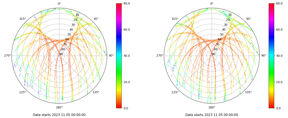
Skyplot for station XIXO. Parameter M1C Data file XIXO00ESP_R_2023309.xtr Skyplot for station XIXO. Parameter M2C Data file XIXO00ESP_R_2023309.xtr
