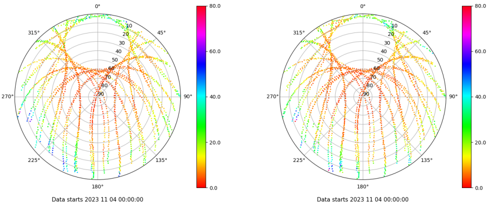
Skyplot for station XIXO. Parameter M1C Data file XIXO00ESP_R_2023308.xtr Skyplot for station XIXO. Parameter M2C Data file XIXO00ESP_R_2023308.xtr
