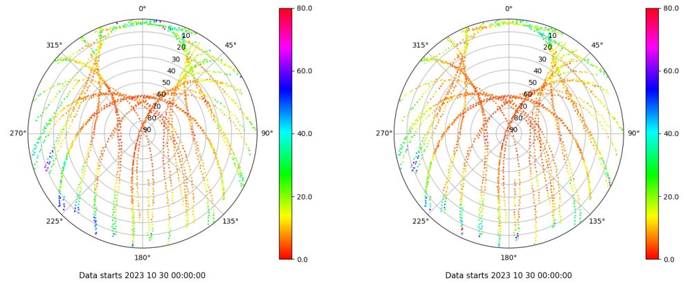
Skyplot for station XIXO. Parameter M1C Data file XIXO00ESP_R_2023303.xtr Skyplot for station XIXO. Parameter M2C Data file XIXO00ESP_R_2023303.xtr
