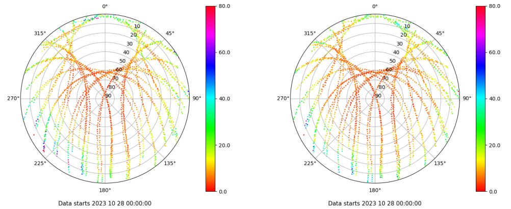
Skyplot for station XIXO. Parameter M1C Data file XIXO00ESP_R_2023301.xtr Skyplot for station XIXO. Parameter M2C Data file XIXO00ESP_R_2023301.xtr
