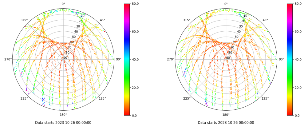
Skyplot for station XIXO. Parameter M1C Data file XIXO00ESP_R_2023299.xtr Skyplot for station XIXO. Parameter M2C Data file XIXO00ESP_R_2023299.xtr
